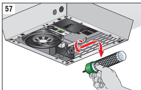
Fig. 57: Atornille suavemente el tubo ionizante sujetándolo por la base ( parte verde ).
