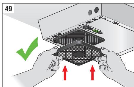
Fig. 49: Vuelva a colocar la tapa del filtro con cierre a presión. Presiónelo sobre la rejilla incorporada en la placa de cierre hasta escuchar el clic del acoplamiento entre las piezas.
