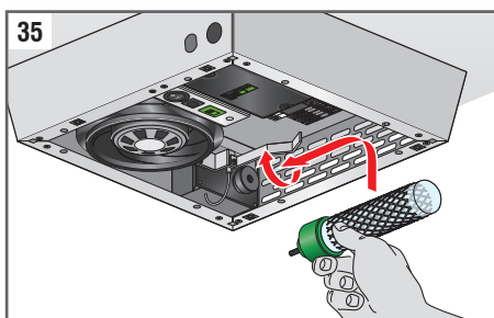
Fig. 35: Atornille suavemente el tubo ionizante sujetándolo por la base (parte verde). Si la operación es difícil, tire ligeramente del soporte de puesta a tierra para que no entre en contacto con la superficie del tubo.
