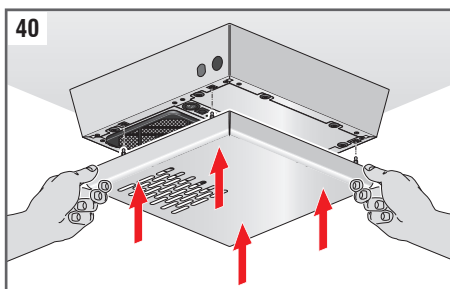
Fig. 40: Vuelva a colocar la cubierta exterior fijándola a los pasadores.
