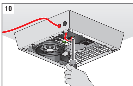
Fig. 10: la tarjeta electrónica puede dar una señal externa para ser conectada a un dispositivo de control y señalización. Si se proporciona, conecte el cable de señal a la tarjeta electrónica. Pase por la carcasa del dispositivo con el prensaestopas especial. Conecte el cable de señal según el diagrama de cableado adjunto.
