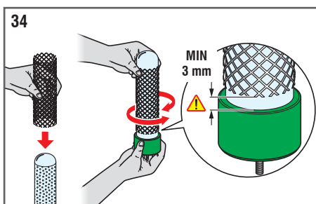
Fig. 34: Vuelva a colocar la malla de metal externa sobre el vidrio del tubo para que se superponga exactamente con la lámina interna.
