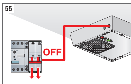
Fig. 55: Desconecte la fuente de alimentación actuando sobre el interruptor magnetotérmico de seguridad situado en el circuito aguas arriba del dispositivo. Asegúrese de que la fuente de alimentación no se pueda restaurar accidentalmente.
