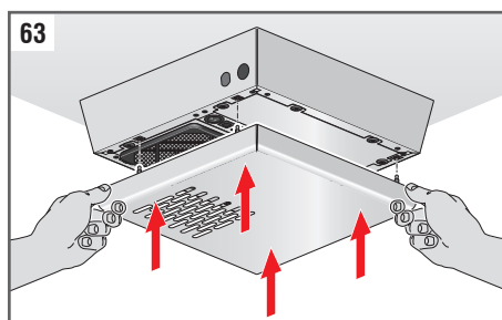
Fig. 63: Vuelva a colocar la cubierta exterior fijándola a los pasadores.
