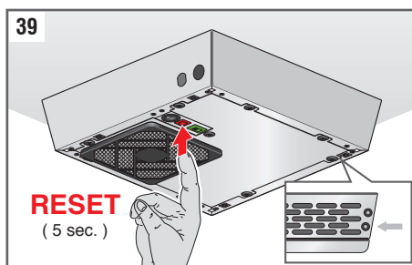
Fig. 39: Mantenga presionado el botón de reset por al menos 5 segundos hasta que se apague el LED de alarma (LED rojo).
