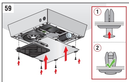
Fig. 59: Vuelva a colocar la placa de cierre atornillando los remaches de plástico de fijación.
