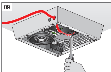
Fig. 09: Conecte el dispositivo a la línea de alimentación. Utilice cable eléctrico de tamaño adecuado.
