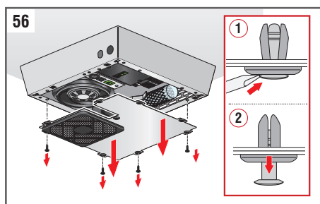
Fig. 56: Retire los remaches de retención de plástico y retire la placa de cierre.
