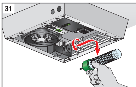
Fig. 31: Atornille suavemente el tubo ionizante sujetándolo por la base (parte verde).
