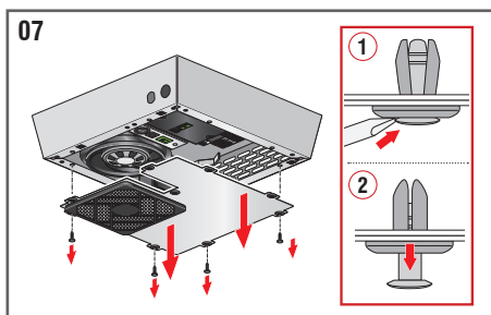
Fig. 07: Retire los remaches de retención de plástico y retire la placa de cierre.
