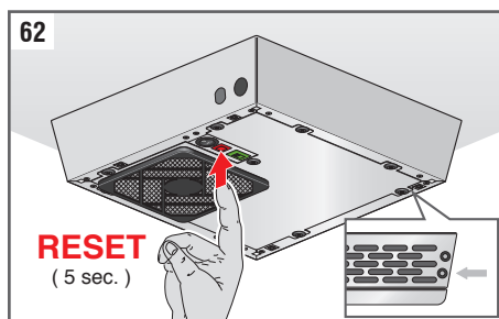
Fig. 62: Mantenga presionado el botón de reset por al menos 5 segundos hasta que se apague el LED de alarma (LED rojo).
