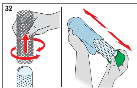
Fig. 32: Retire la malla exterior del tubo: si la operación es difícil, gire ligeramente la malla alrededor del vidrio.
