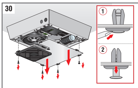
Fig. 30: Retire los remaches de retención de plástico y retire la placa de cierre.
