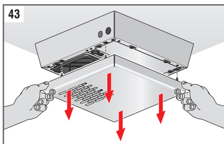
Fig. 43: Retire la cubierta externa agarrándola por un lado y tirando para desengancharla del dispositivo.
