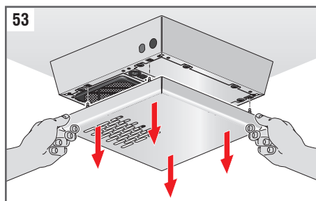
Fig. 53: Retire la cubierta externa que está fijada con pasadores de enclavamiento. Tire mientras agarra, lateralmente, la cubierta para quitarla.
