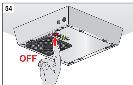
Fig. 54: Apague el dispositivo usando el interruptor 0 / I, llevándolo a la posición 0.
