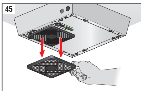
Fig. 45: Retire la tapa del filtro presionando los lados y tirando de ella hacia usted.
