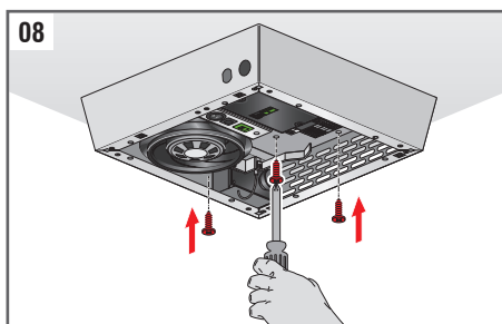
Fig. 08 Fije el dispositivo al techo o a la pared usando los tres orificios provistos. Elija el sistema de fijación adecuado al tipo de techo o de pared.
