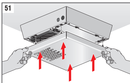
Fig. 51: Vuelva a colocar la cubierta exterior fijándola a los pasadores.
