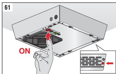
Fig. 61: Gire el interruptor a ON para verificar la presencia de voltaje en el dispositivo. Verificar el funcionamiento del dispositivo, se debe escuchar un leve chisporroteo proveniente del tubo ionizante y se percibirá el flujo de aire generado por el ventilador.
