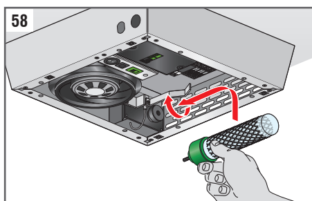
Fig. 58: Atornille suavemente el tubo ionizante sujetándolo por la base (parte verde). Si la operación es difícil, tire ligeramente del soporte de puesta a tierra para que no entre en contacto con la superficie del tubo.
