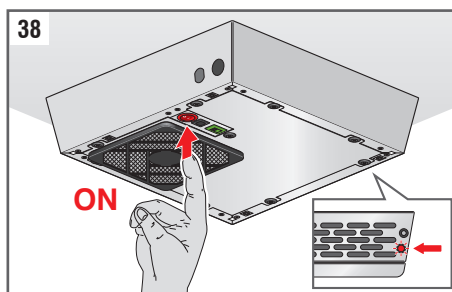
Fig. 38: Gire el interruptor a ON para verificar la presencia de voltaje en el dispositivo. Verificar el funcionamiento del dispositivo, se debe escuchar un leve chisporroteo proveniente del tubo ionizante y se percibirá el flujo de aire generado por el ventilador.
