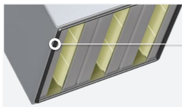
Fig. 20 : Positionner les filtres propres/neufs. Poussez les languettes de blocage du filtre vers l'intérieur jusqu'à ce que vous entendiez un déclic. S'assurer que le joint en caoutchouc du filtre soit tourné vers le bas.
