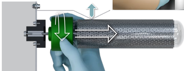
Fig. 28 : Dégager le treillis à l'extérieur du tube. Si l'opération est difficile, tourner le treillis autour du verre.
