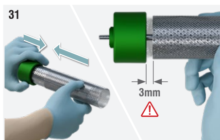
Fig. 31 : Replacer le treillis métallique externe sur le verre du tube de manière à ce qu'il se superpose exactement à la tôle à l'intérieur.
