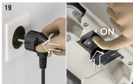
Fig. 19 : Reconnecter la fiche d'alimentation. Allumer le dispositif d'ionisation en amenant l'interrupteur On/Off dans la position I.
