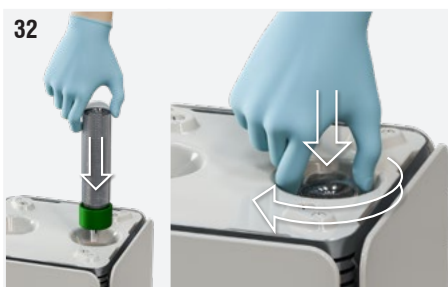
Fig. 32: Positionner le nouveau tube ionisant dans l' emplacement en agissant toujours sur la surface en verre accessible avec la main depuis les fentes.
