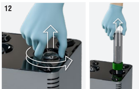
Fig. 12: Svitare delicatamente il tubo ionizzante agendo sulla superficie di vetro raggiungibile a mano dalle apposite fessure.
