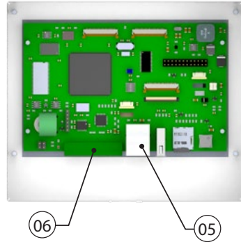
VISTA POSTERIORE
