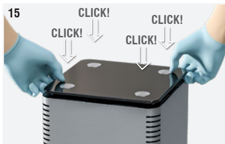
Fig. 15: Vuelva a colocar la cubierta en el dispositivo empujándola hasta que sienta que las partes están enganchadas.
