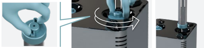
Fig. 13: Limpiar el tubo con un paño ligeramente húmedo (que no suelte fibras), girando ligeramente la malla metálica alrededor del cristal.
