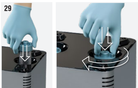
Fig. 29: Vuelva a colocar los nuevos tubos ionizantes en su asiento atornillándolos, trabajando siempre en la tapa de seguridad.
