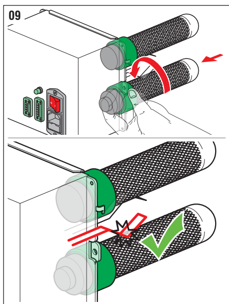
Fig. 09: Riavvitare delicatamente il tubo ionizzante afferrandolo alla base (parte verde).
