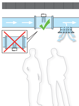
APPLICAZIONE SUPERIORE SU CONDOTTO ORIZZONTALE
