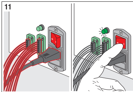
Fig. 11: Reinserire la spina d'alimentazione e tutte le altre spine nelle apposite prese del modulo JONIX VMC. Accendere il modulo premendo il pulsante di On/Off portandolo nella posizione I. Verificare il funzionamento del dispositivo, deve essere udibile un leggero sfrigolio proveniente dai tubi.
