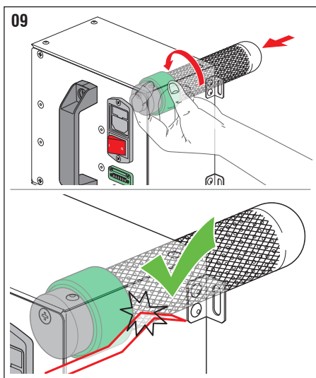
Fig. 09: Riavvitare delicatamente il tubo ionizzante afferrandolo alla base (parte verde).
