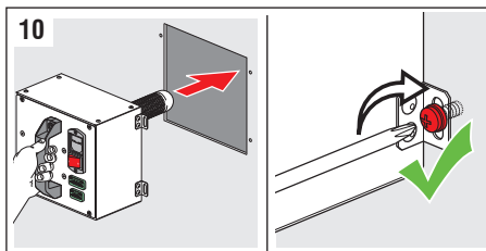
Fig. 10: Riposizionare il dispositivo JONIX duct inserendo orizzontalmente i tubi ionizzanti nell'apposito foro attraverso la sua maniglia ed avvitare le 4 viti che fissano le staffe alla parete.
