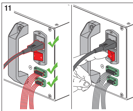
Fig. 11: Reinserire la spina d'alimentazione e tutte le altre spine nelle apposite prese del modulo JONIX duct.
